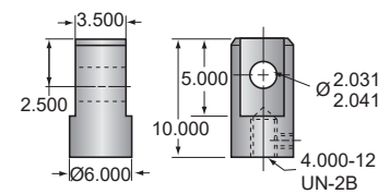
Clevis end (optional) 75-MSJ
