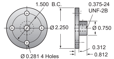
Top plate (optional) 0.5-BSJ / 0.5HL-BSJ
