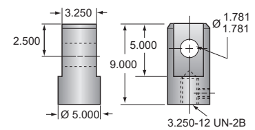
Clevis end (optional) 50-BSJ
